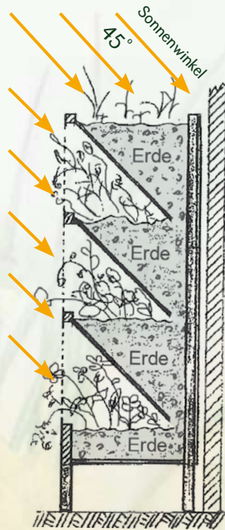
Kräutermax in Schnittansicht ▲
